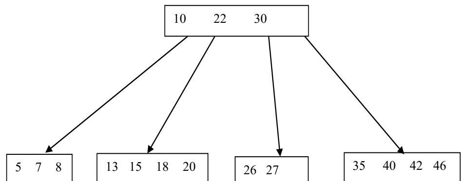
Step 3
