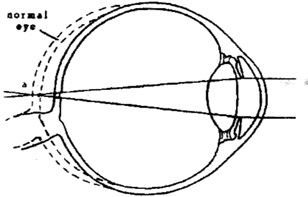
Fig. 2.1 Hyperopia (Farsightedness)
